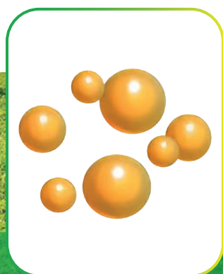
Timolo e Geraniolo
