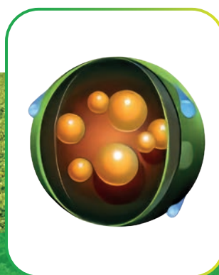
Incapsulazione in soluzione acquosa
