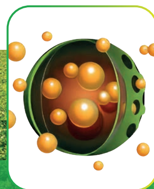
Rilascio dei terpeni dopo l'applicazione
