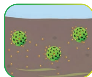
Quando il terreno si bagna nuovamente, i pori si riaprono, rilasciando i terpeni rimanenti
