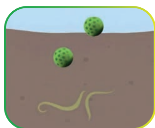
Il prodotto liquido contenente i terpeni incapsulati viene applicato sul terreno umido
