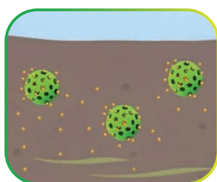
Il contatto con il terreno bagnato fa aprire i pori delle capsule che rilasciano i terpeni che entrano in contatto con i nematodi
